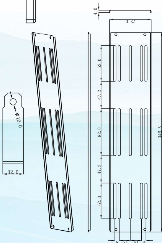
电源板孔位
