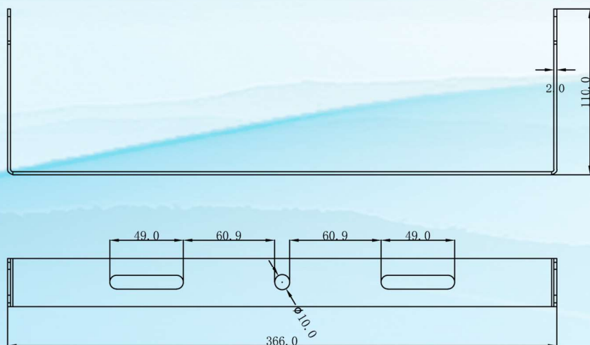
支架孔位
