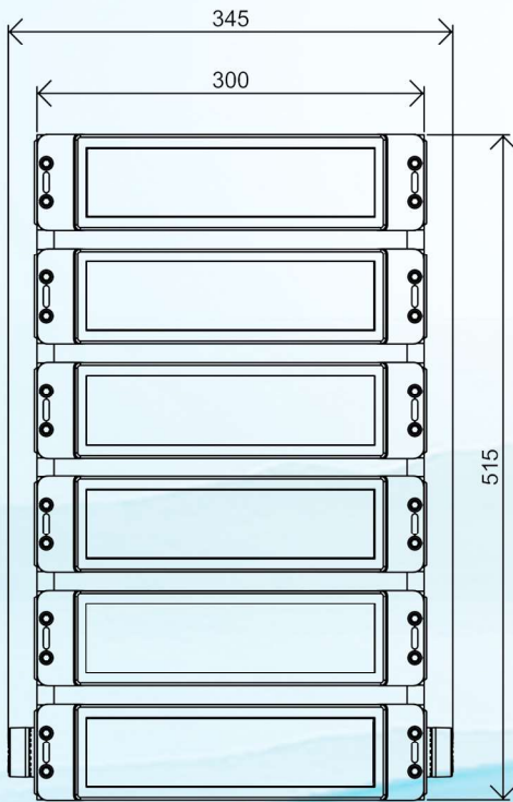
主视图
